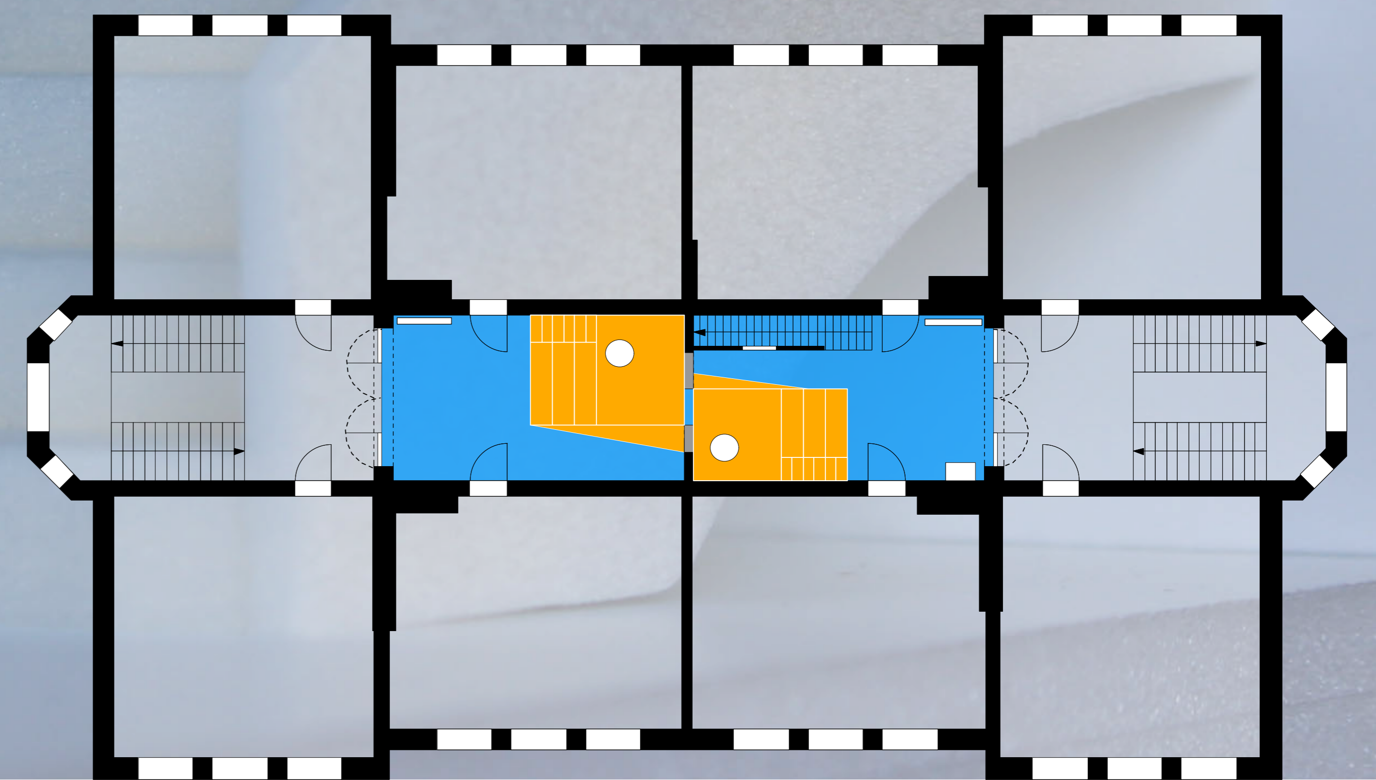
Obergeschoss 2
